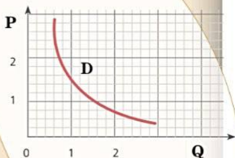
КРИВАЯ СПРОСА
